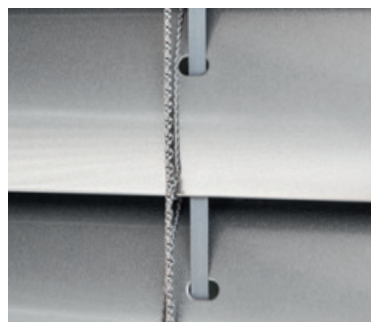
Felhúzószálas lyukasztás
