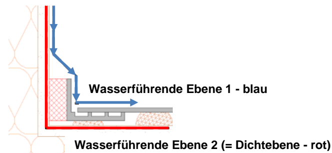
Abbildung 4: Beispiel für den Anschluss der Fensterbank an die Laibung mit zwei wasserführenden Ebenen (Ebene 1 entspricht der Fensterbank; Ebene 2 entspricht der wannenförmigen Abdichtung)
