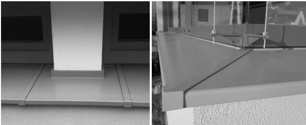
Abbildung 8: Fensterbank mit Stoßverbinder und Eckausführung
